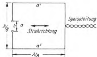
Bild 1. Dipol-Richtantenne mit abgelenkten Strahlenden und zweiseitiger Strahlung.
