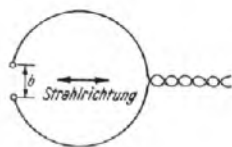
Links: Bild 3. Kreisförmig gebogene Dipol-Richtantenne nach Reinartz.
